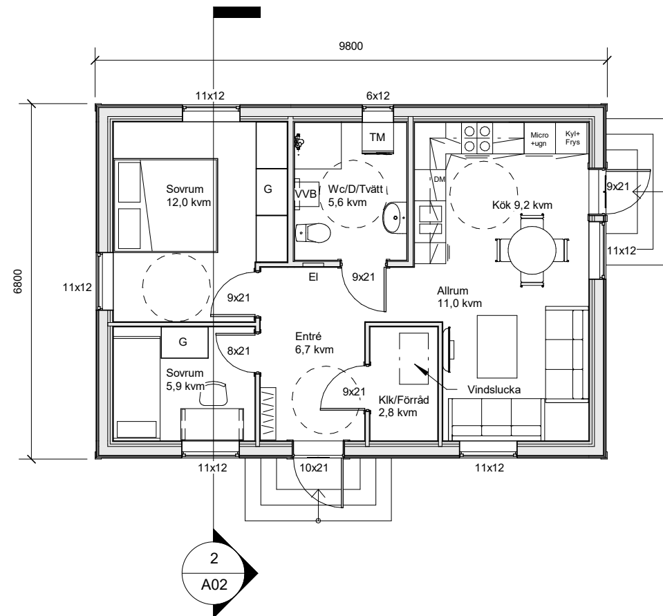
1 Plan 1 : 100
